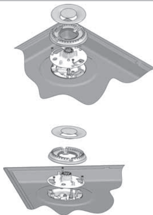
VISTA DE DESPIEZO DEL QUEMADOR
